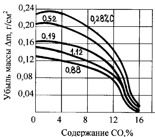
Рис.1.3. Влияние содержания СО в атмосфере печи на скорость коррозии углеродистых сталей при температуре 1260°С (выдержка 40 мин).
