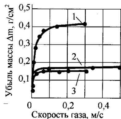
Рис.1.4. Влияние скорости движения газовой среды на кинетику коррозии стали с 0,15%С при температуре 1260°С (выдержка 40 мин): 1 - пары воды, 2-воздух, 3-углекислый газ.
