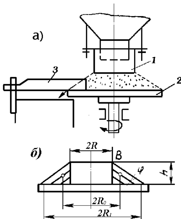
Рис. 2. Схема к расчету тарельчатого питателя: 1–телескопический патрубок; 2–диск; 3–скребок
