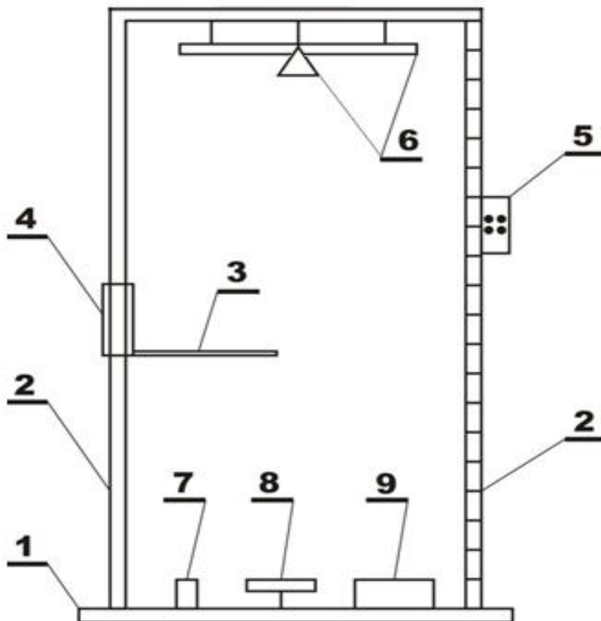
Рис. 1. Схема внешнего вида осветительной установки
